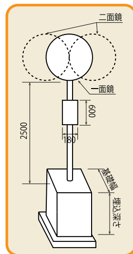
【標準設置図 単位：mm】
