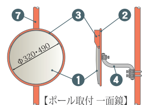
【ポール取付 一面鏡】
