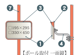
【ポール取付 一面鏡】
