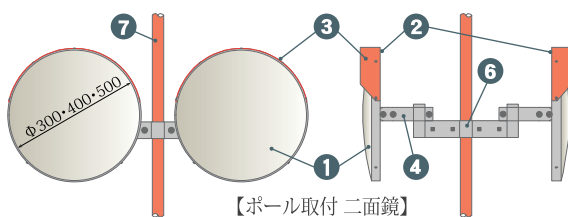
【ポール取付 二面鏡】
