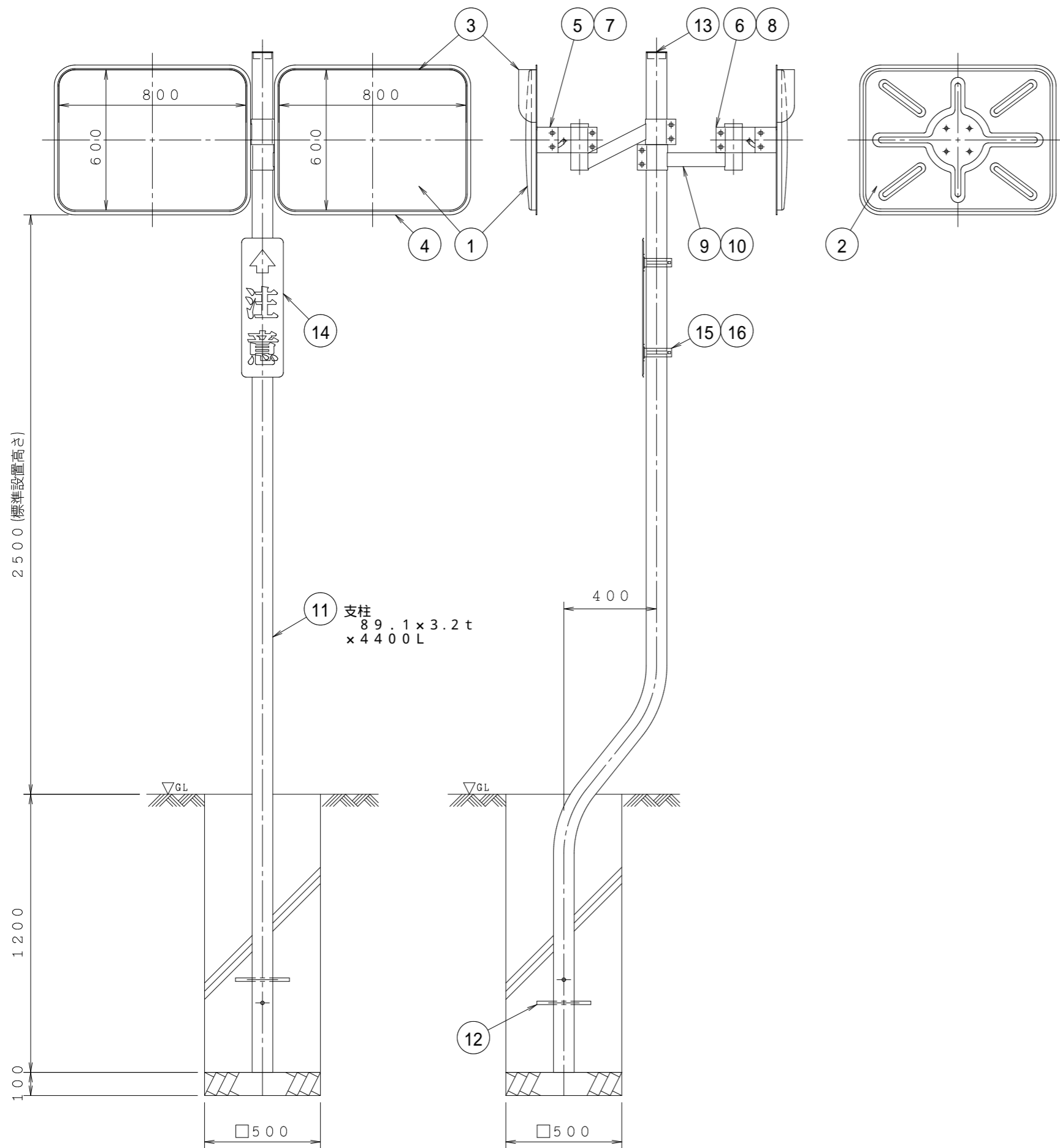
正面図
