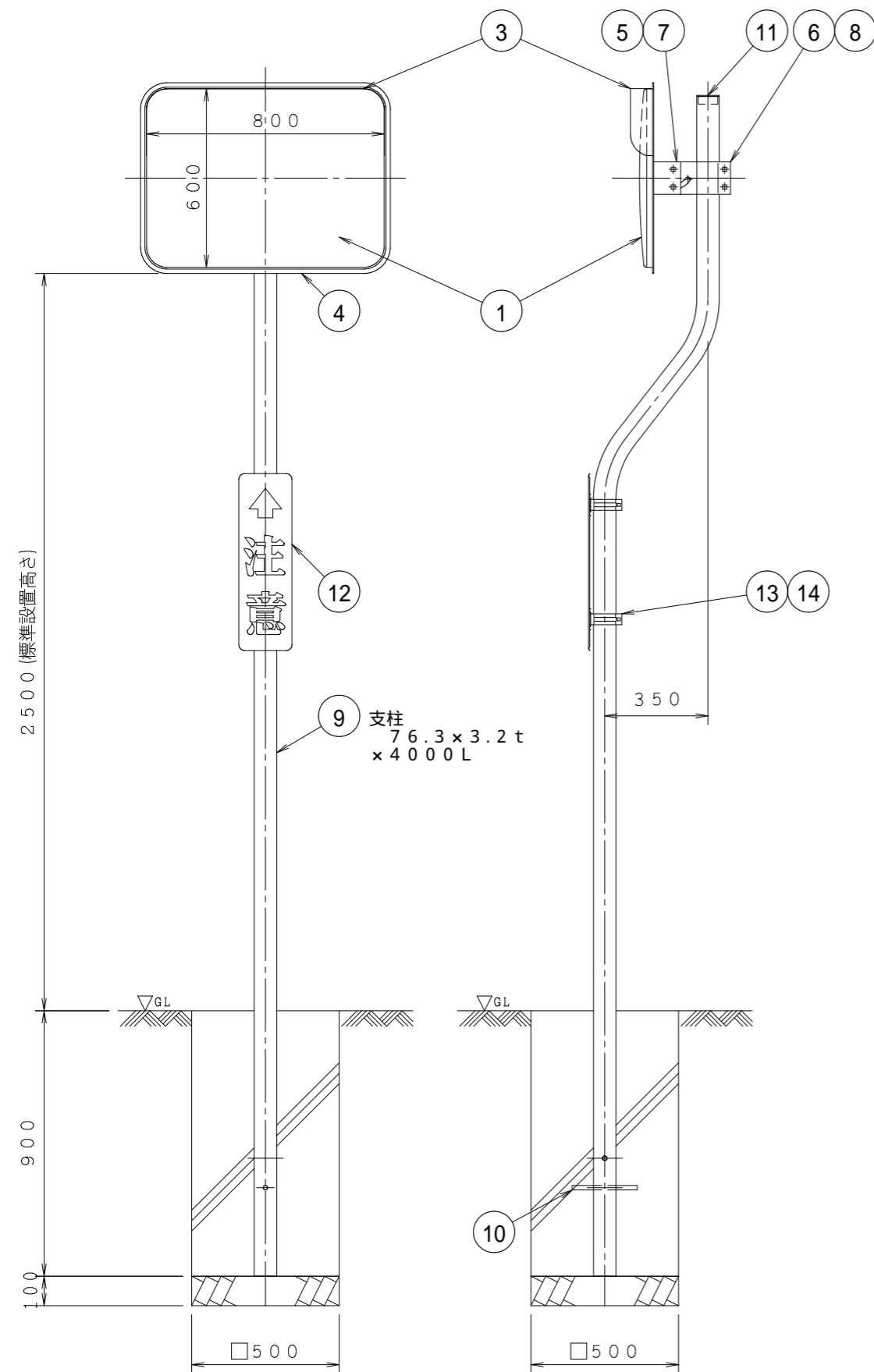
正面図
