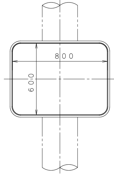
正面図
