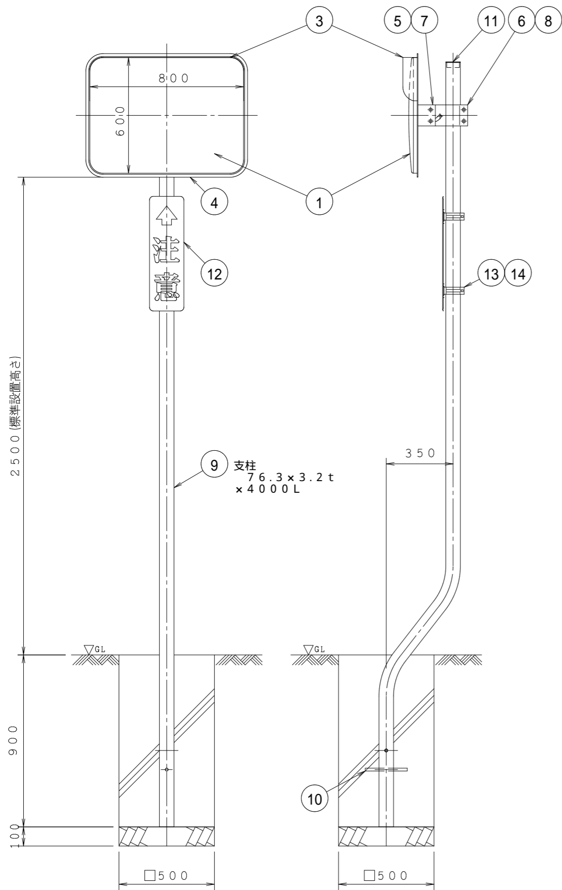
正面図
