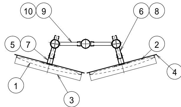
平面視図
