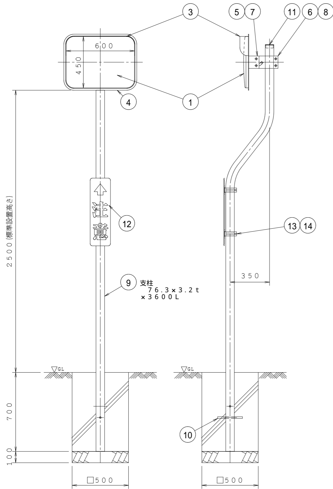
正面図
