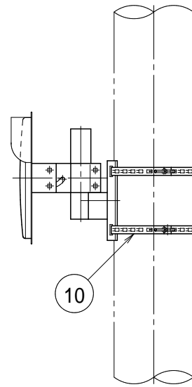
側面図
