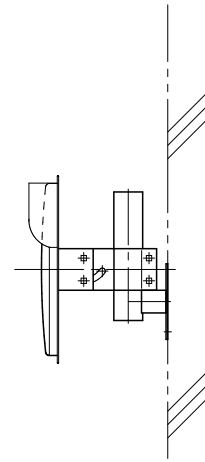
側面図
