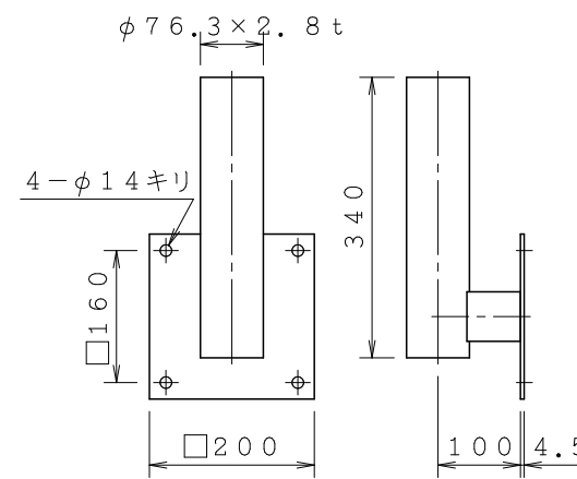
9 壁面取付金具 (S=1/10)
