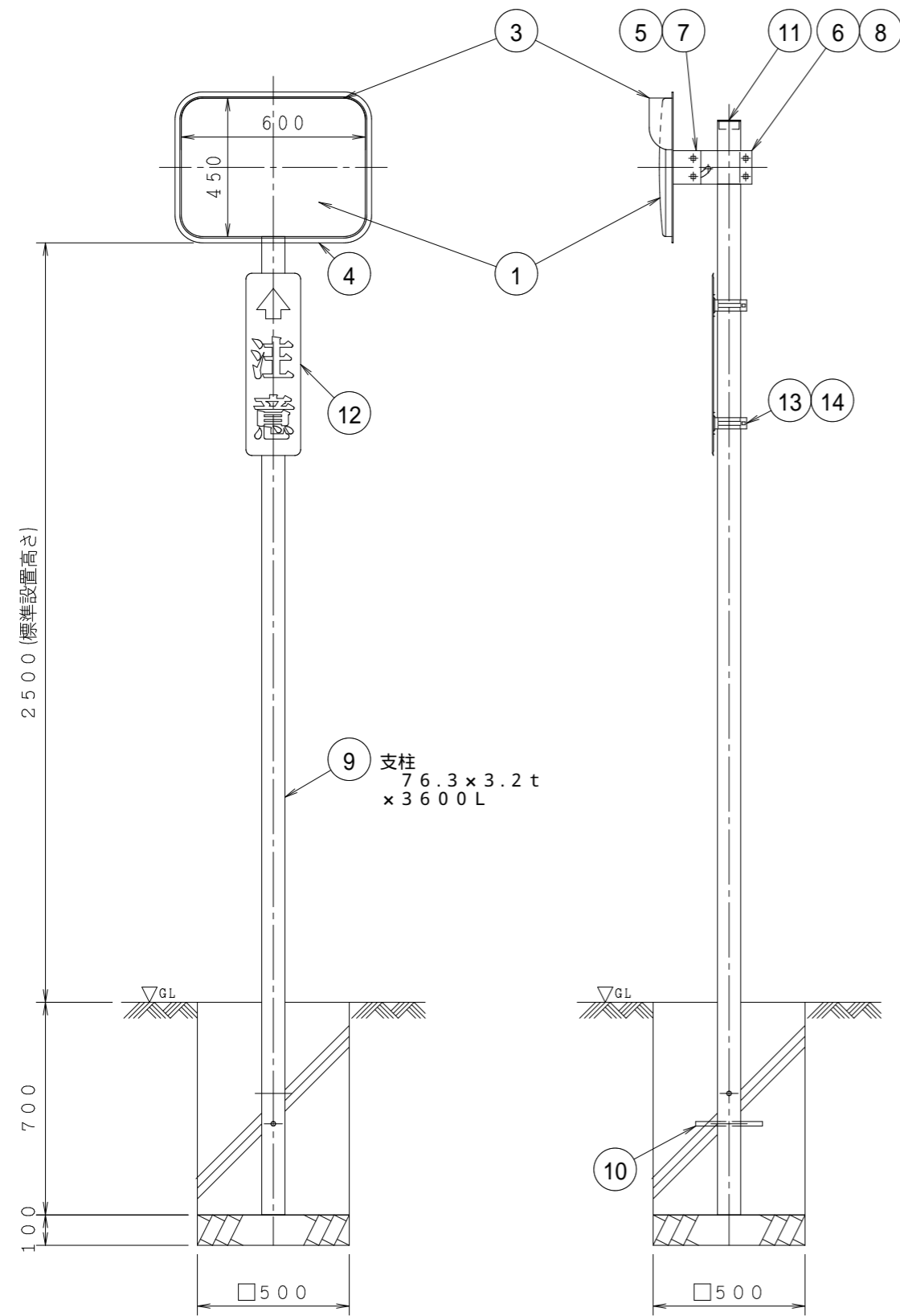
正面図
