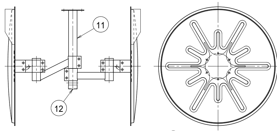
2 バックプレート (S=1/20)
