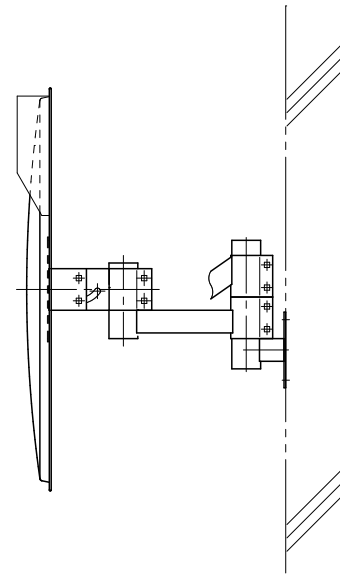
側面図
