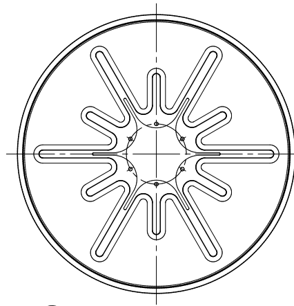
② バックプレート (S=1/20)
