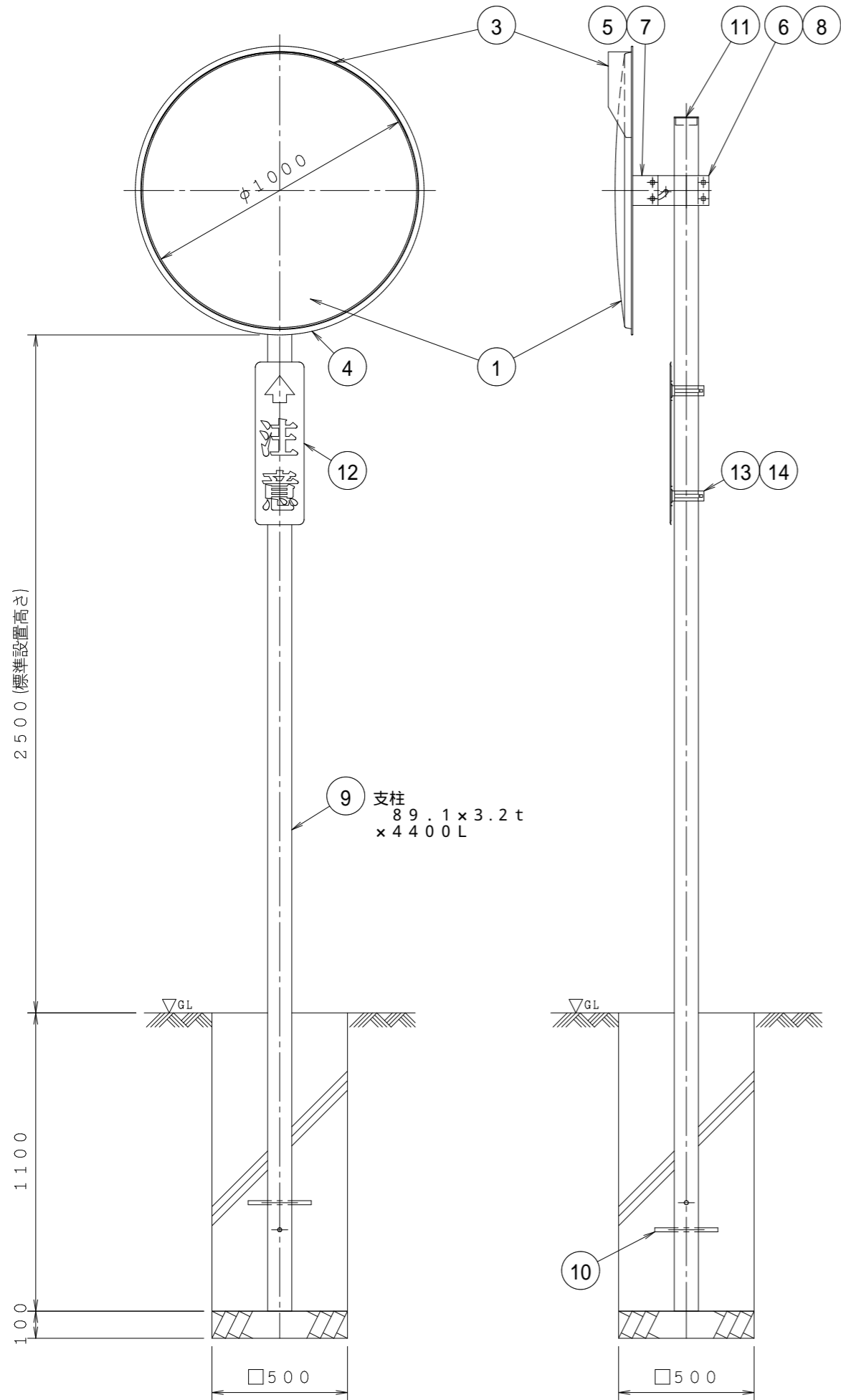
正面図
