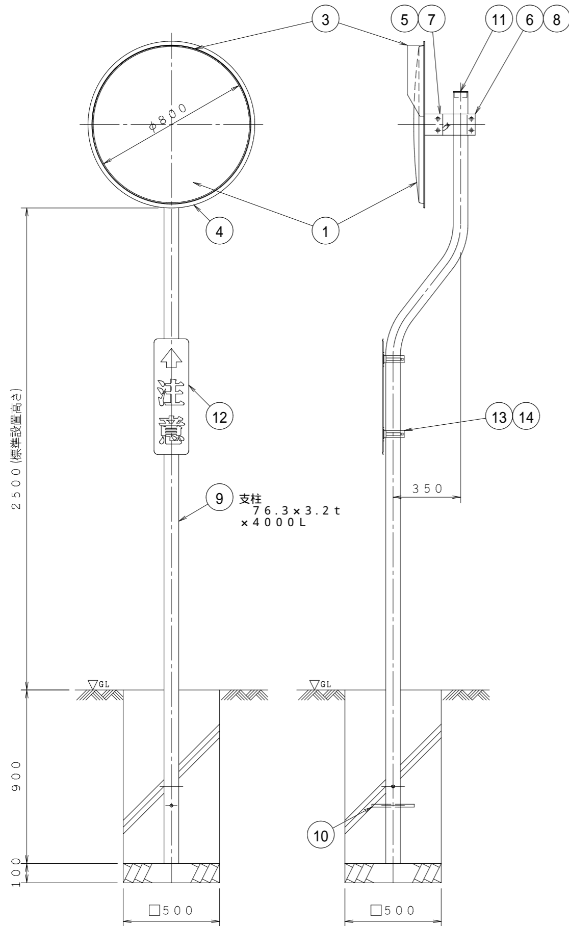
正面図
