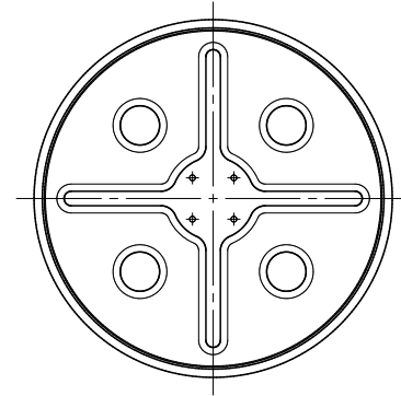
2 バックプレート (S=1/20)
