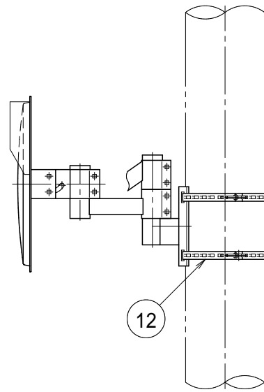
側面図
