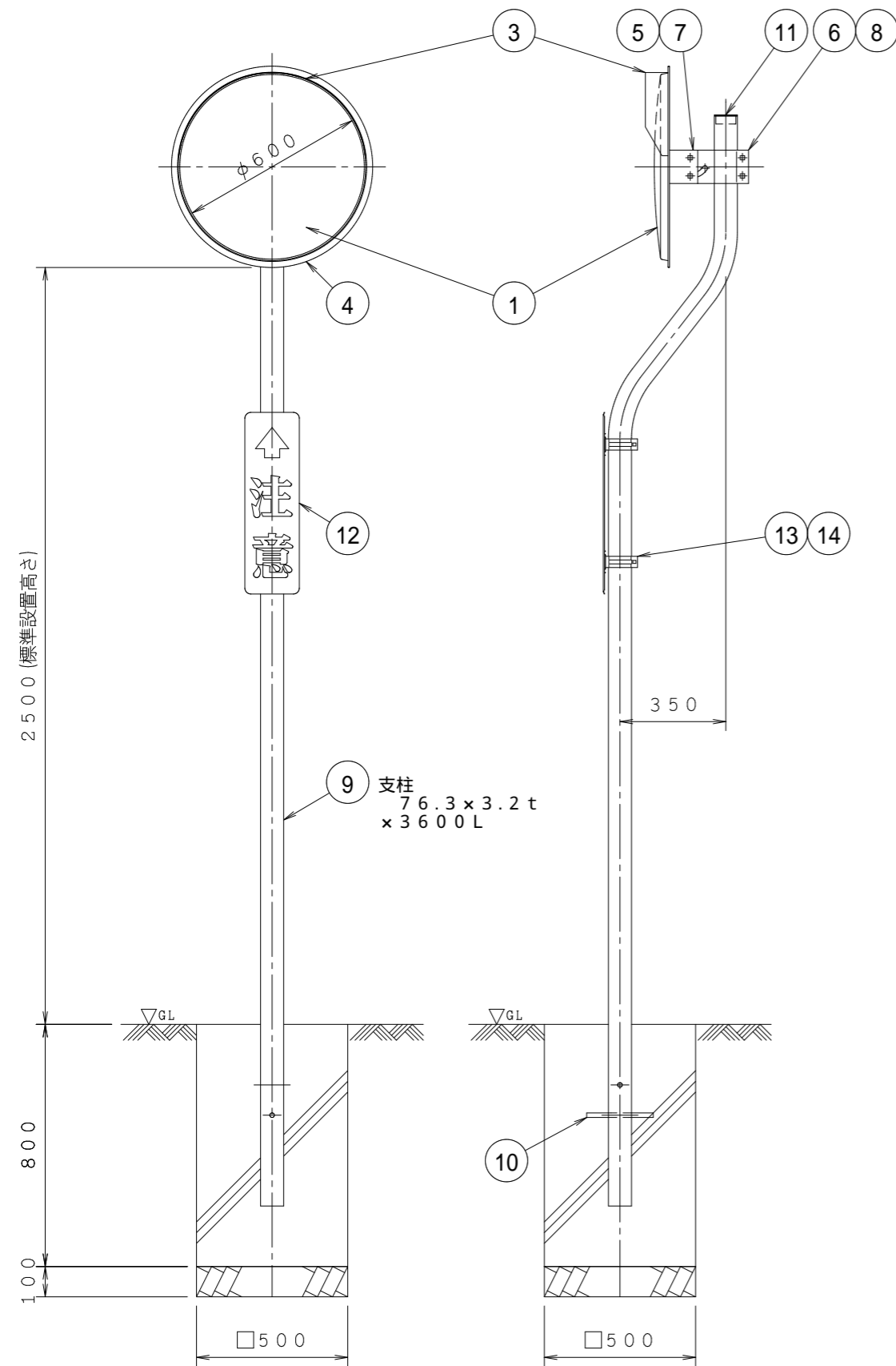
正面図
