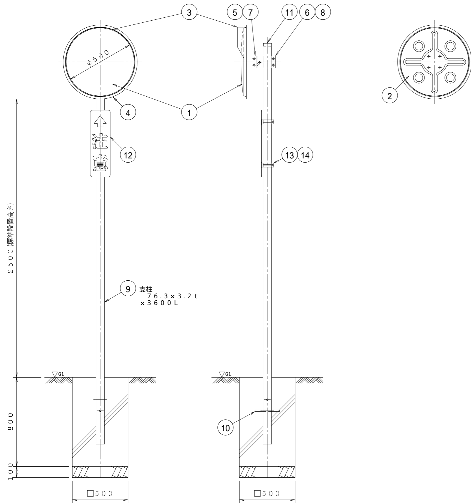
正面図
