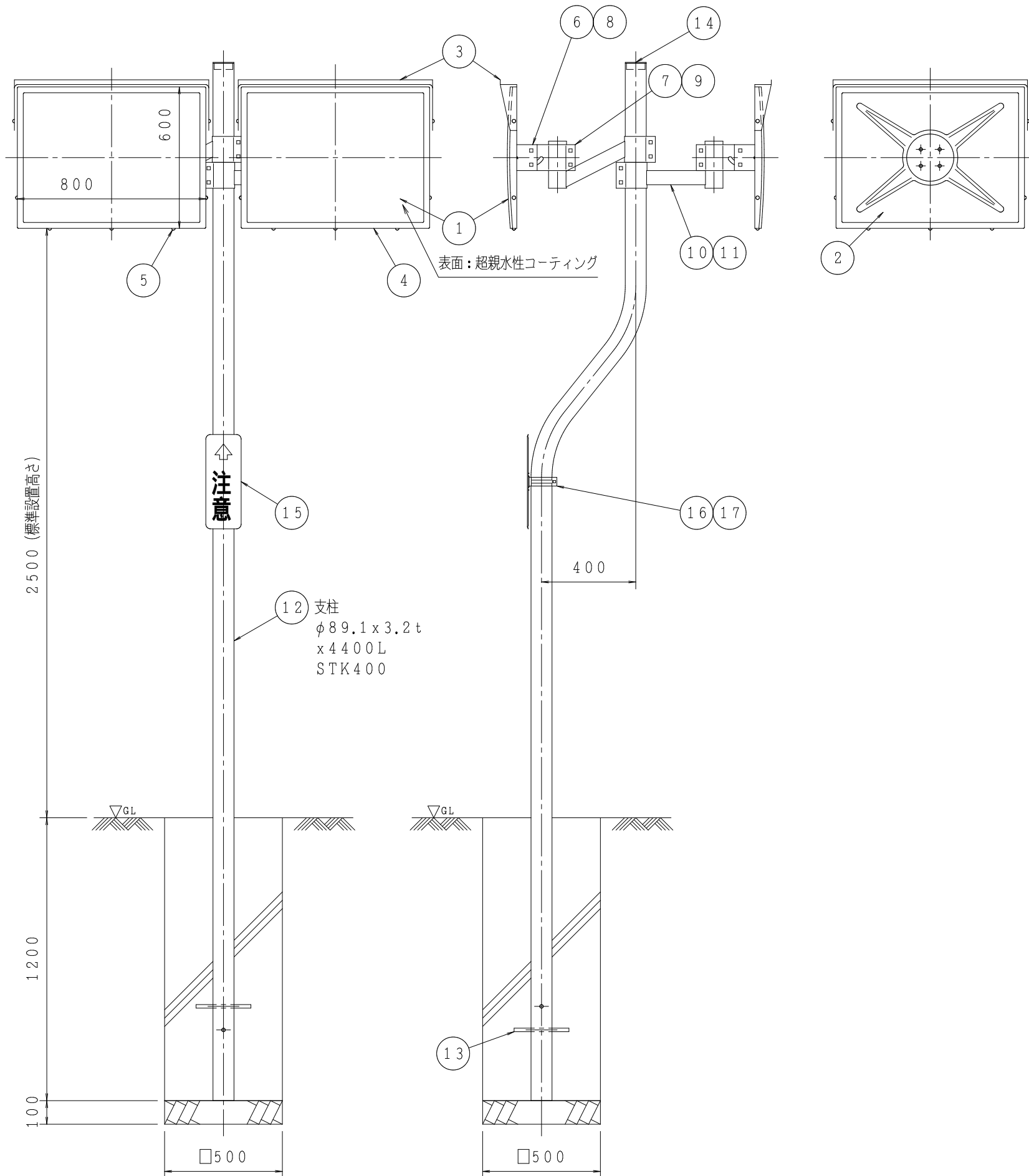
正面図
