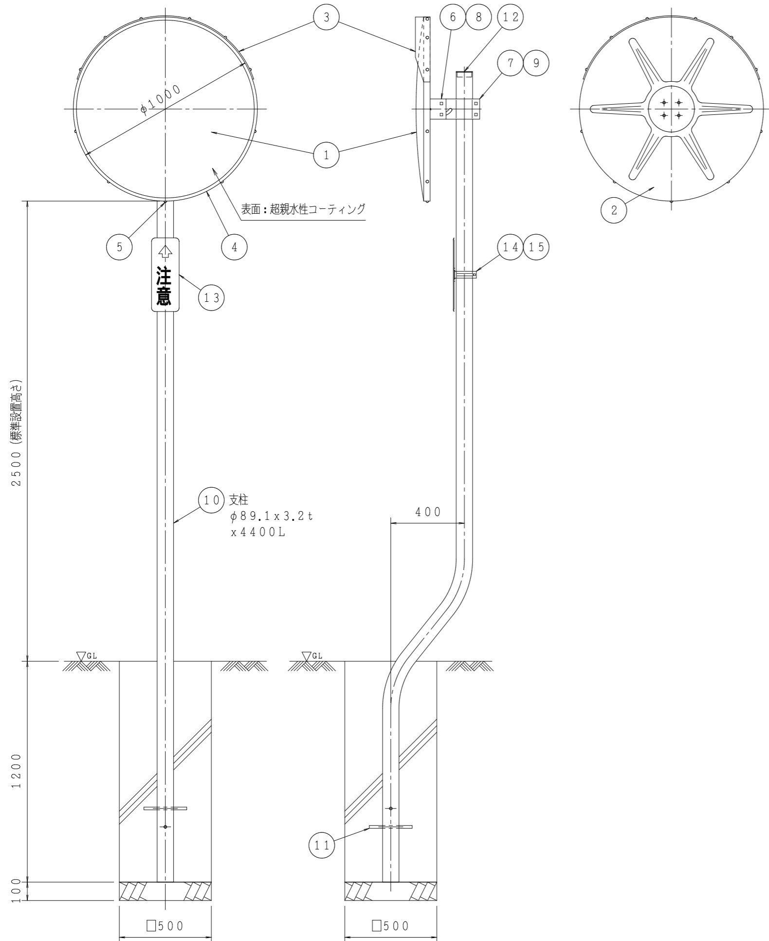
正面図
