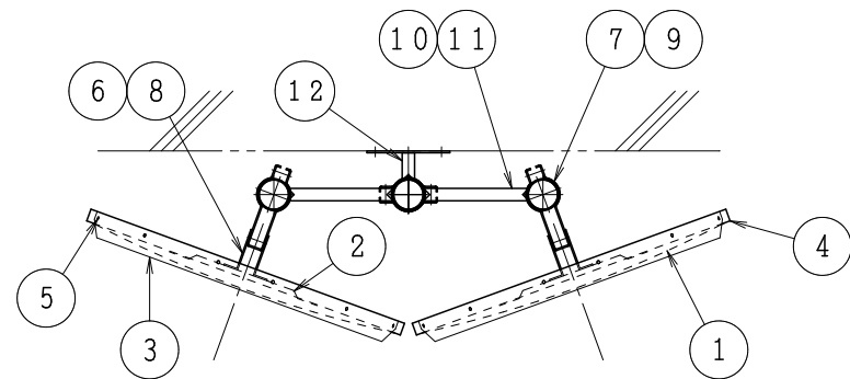
平面視図
