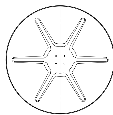
② バックプレート (S=1/20)
