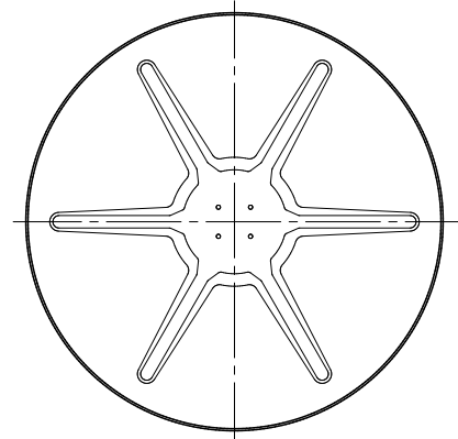
2) バックプレート (S=1/20)
