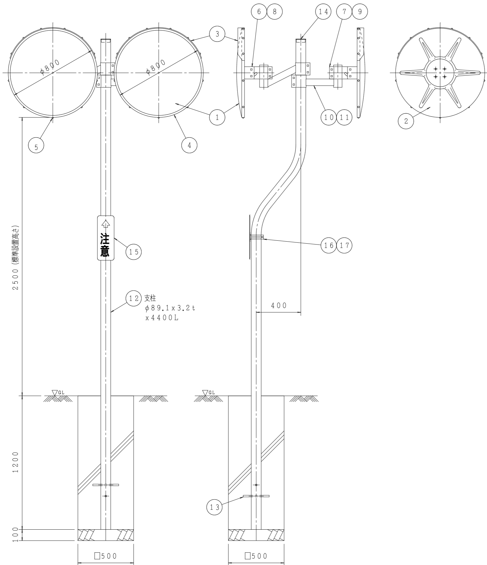
正面図
