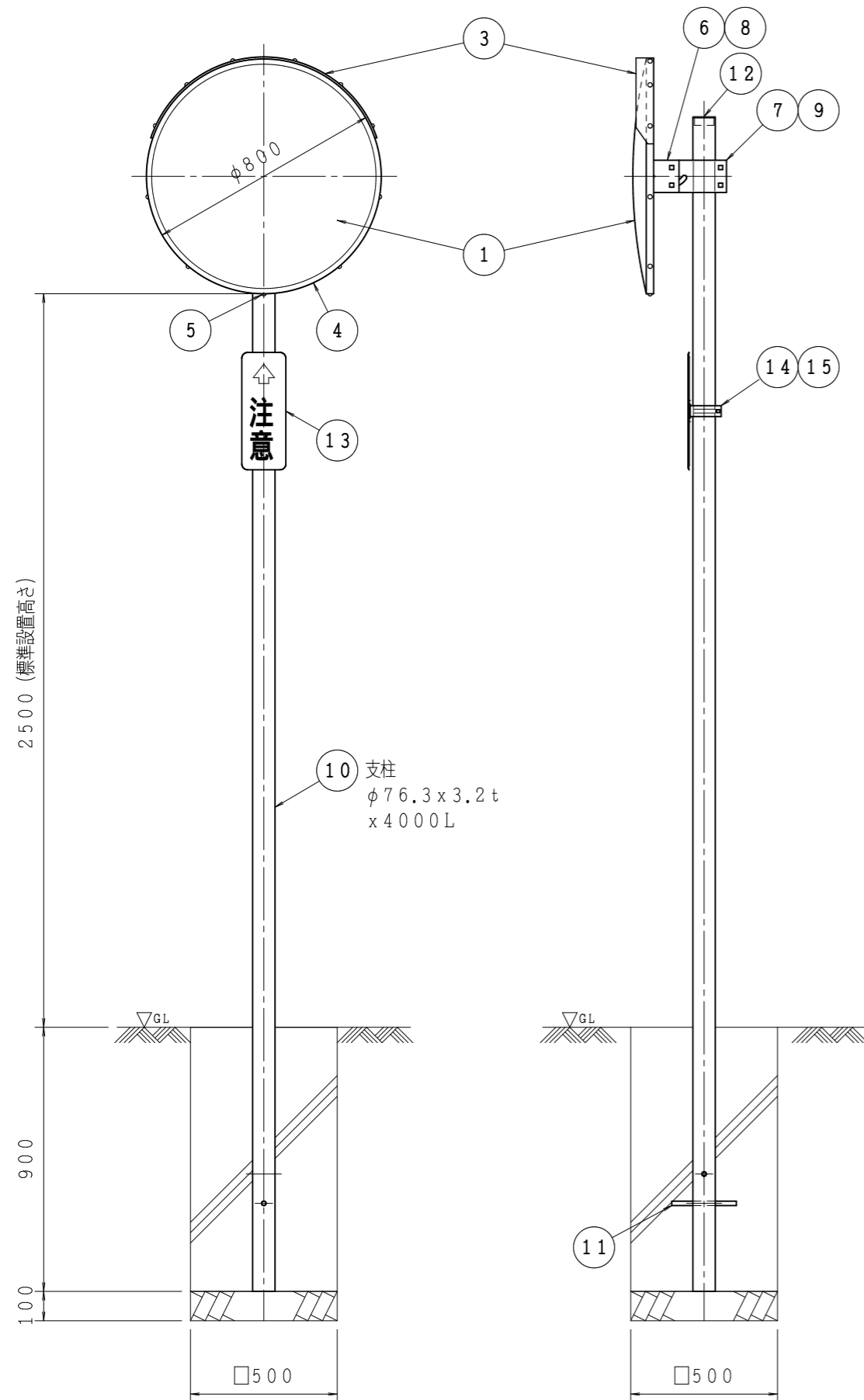
正面図
