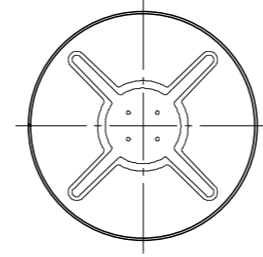
2 バックプレート (S=1/20)
